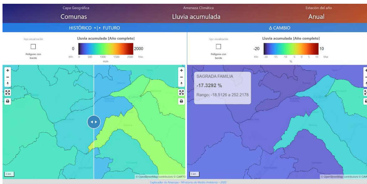
Figura 12. Lluvia acumulada
