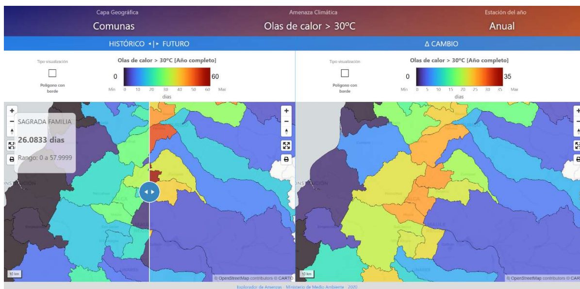
Figura 10. Olas de calor mayores a 30°
