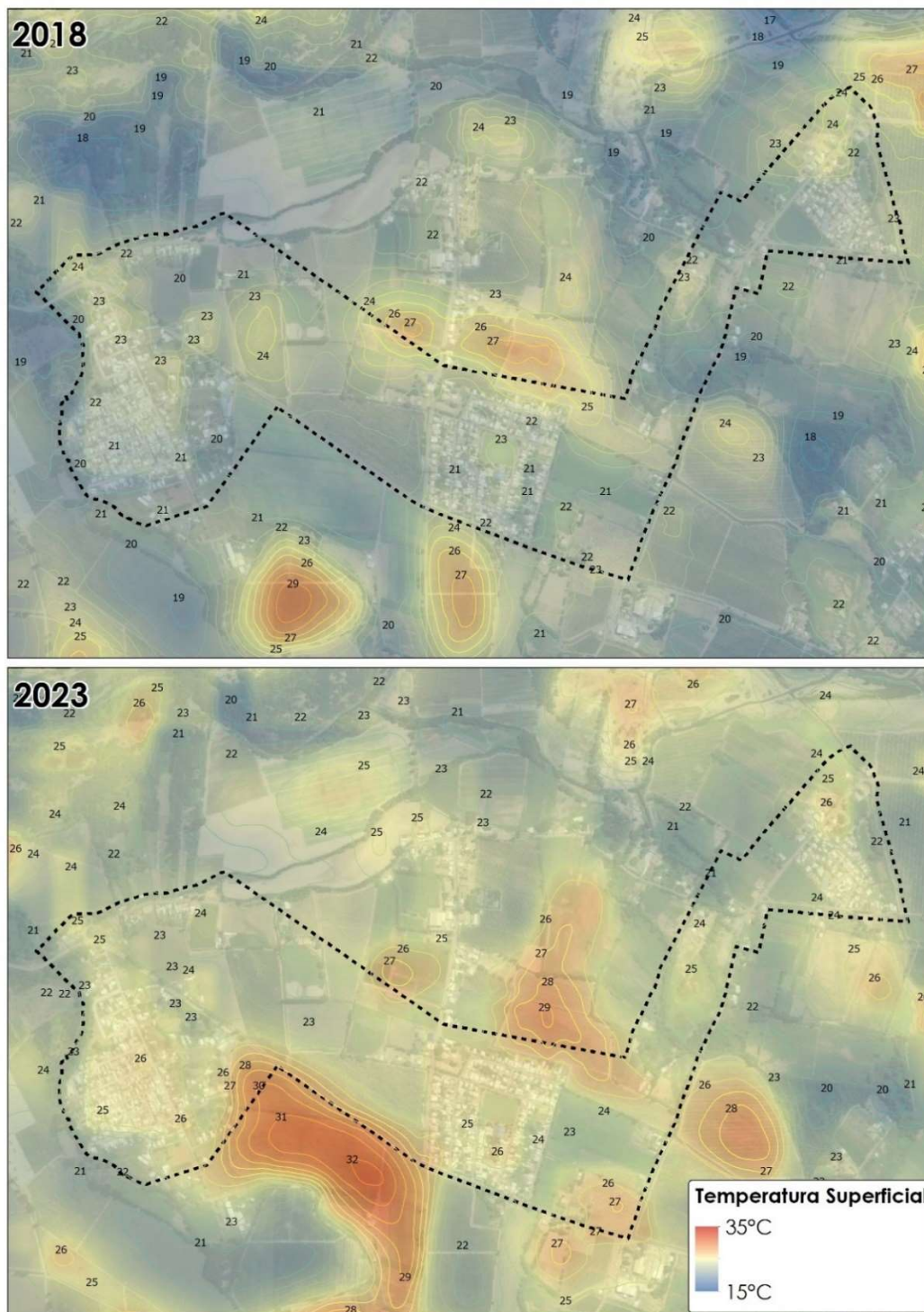
Figura 46. Presencia de suelo urbano afectado por Polos de calor, Lo Valdivia
