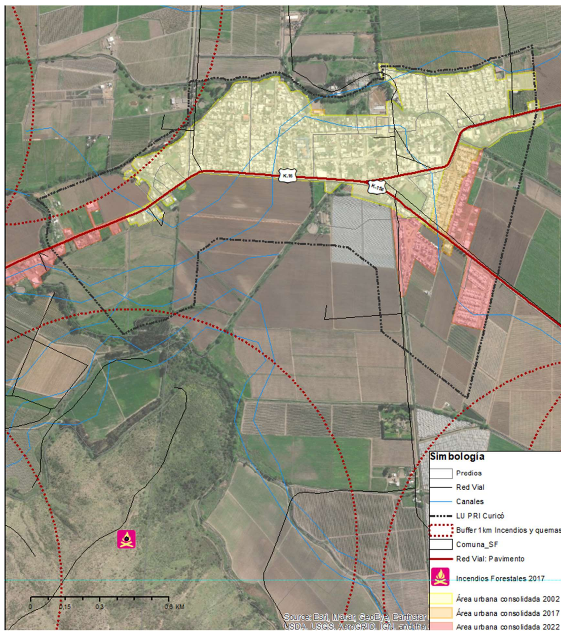
Figura 40. Presencia de suelo urbano afectado por Incendios Forestales, Sagrada Familia
