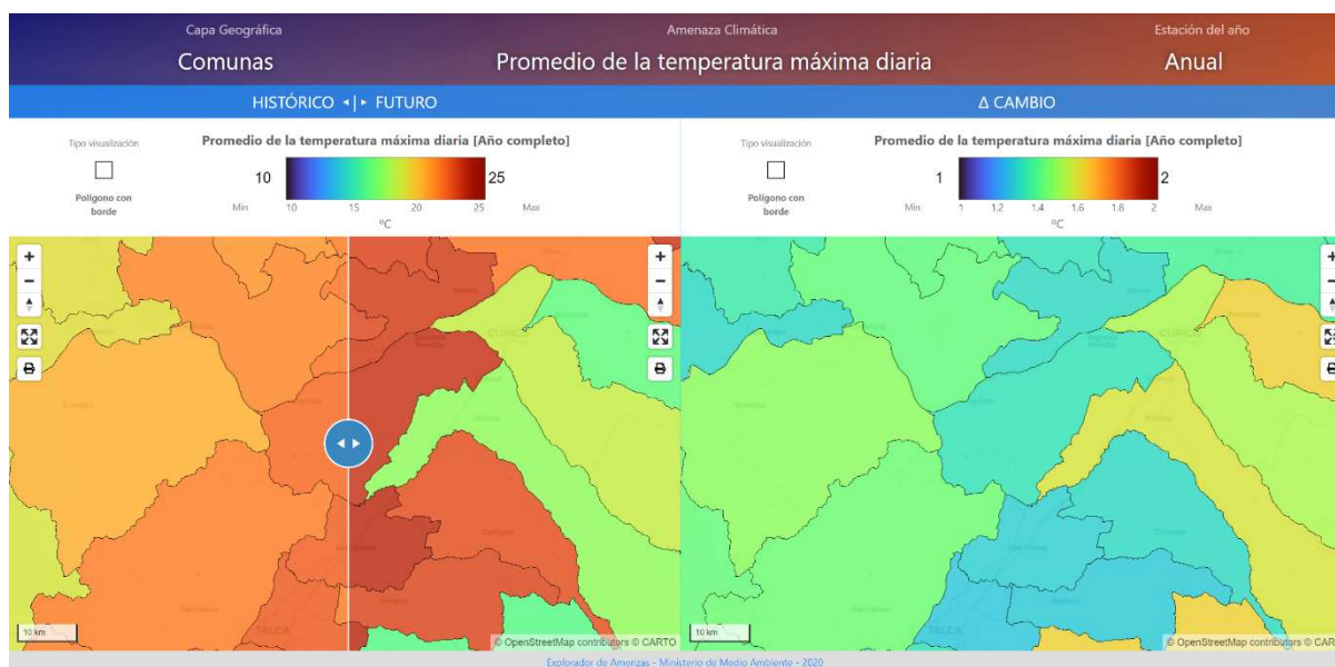
Figura 9. Promedio de la temperatura máxima diaria
