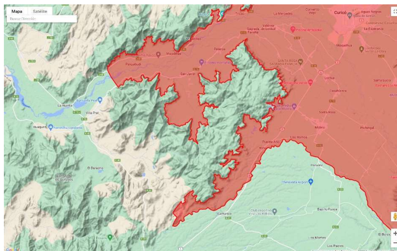
Figura 19. Zona Saturada por MP 2,5
