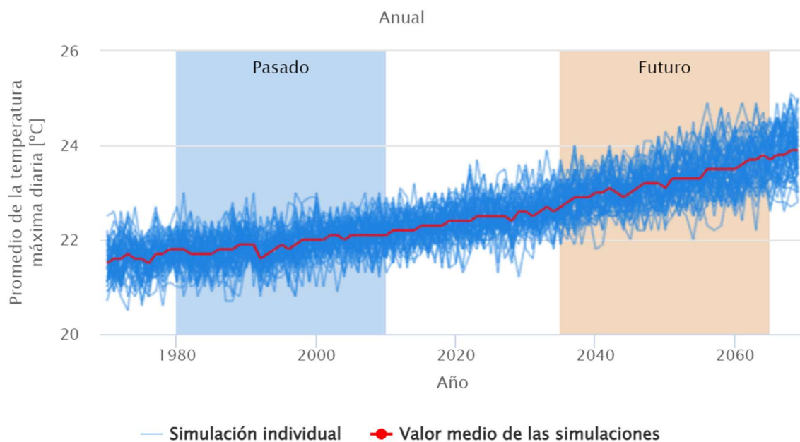
Figura 8. Promedio de la temperatura máxima diaria
