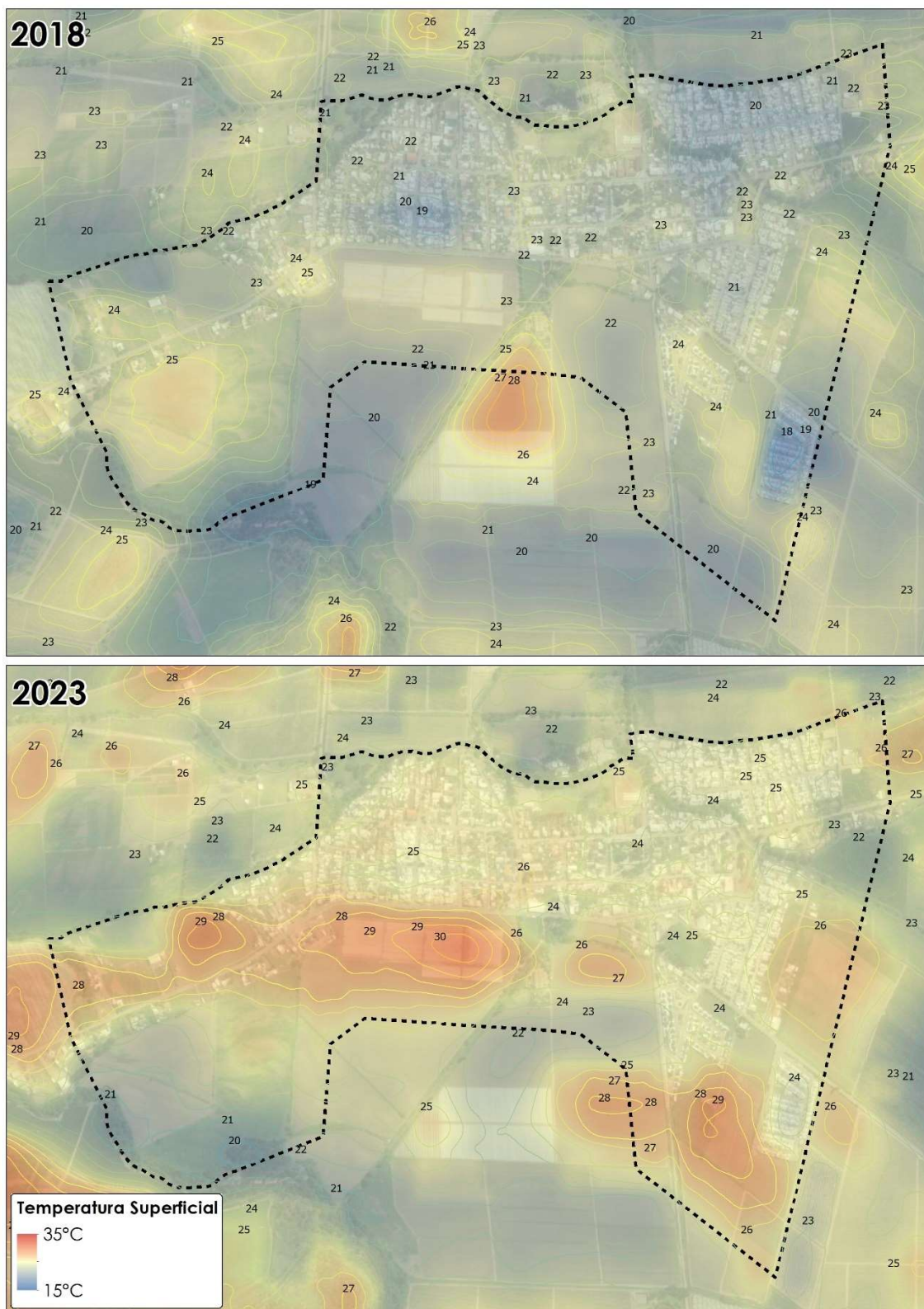
Figura 45. Presencia de suelo urbano afectado por Polos de calor, Sagrada Familia
