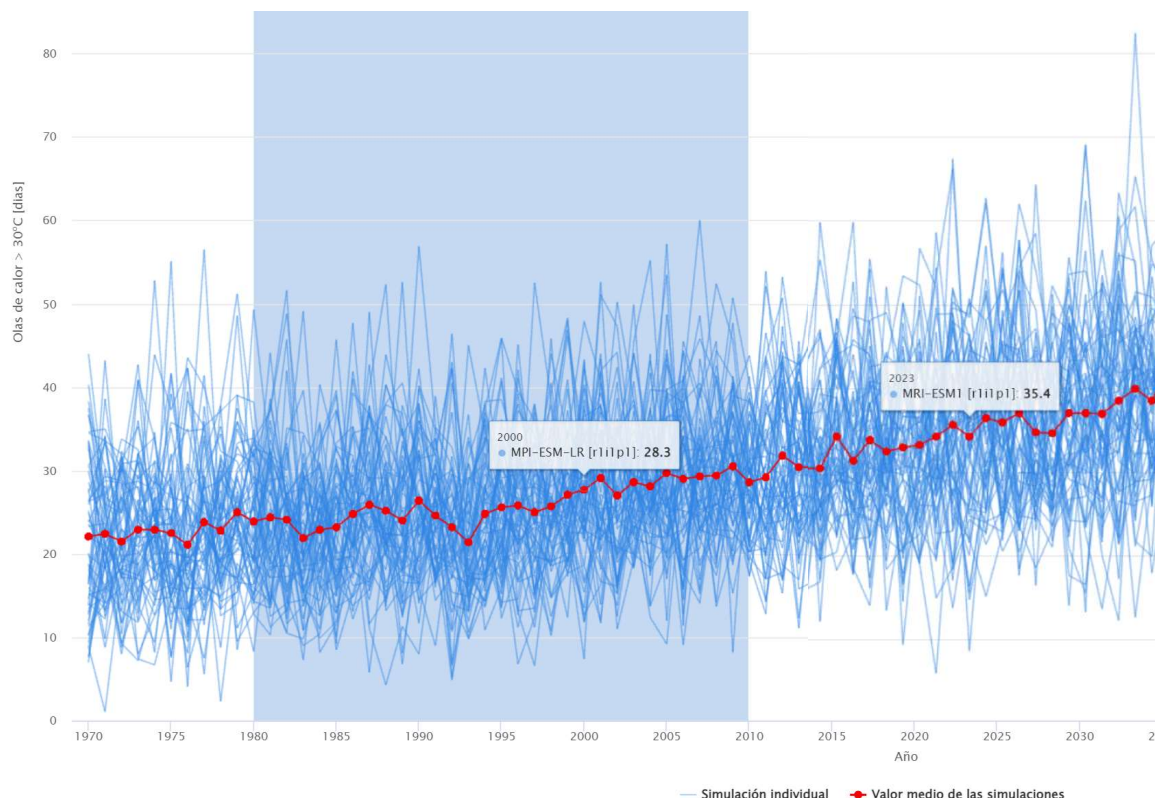
Figura 44. Afectación por Olas de Calor (días con temperaturas mayores a 30°C)
