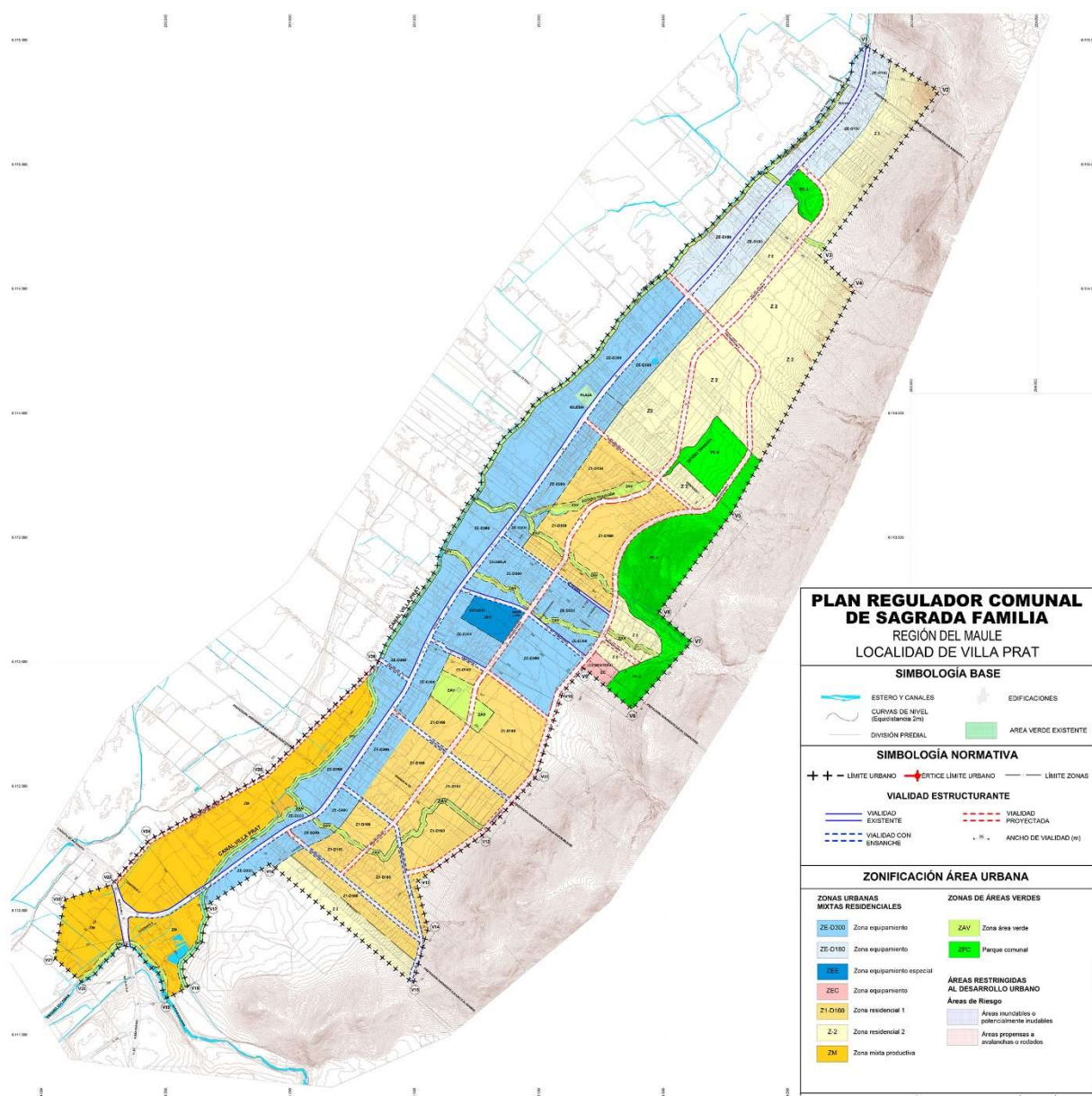
Figura 84. Opción de Desarrollo para Anteproyecto, Villa Prat
