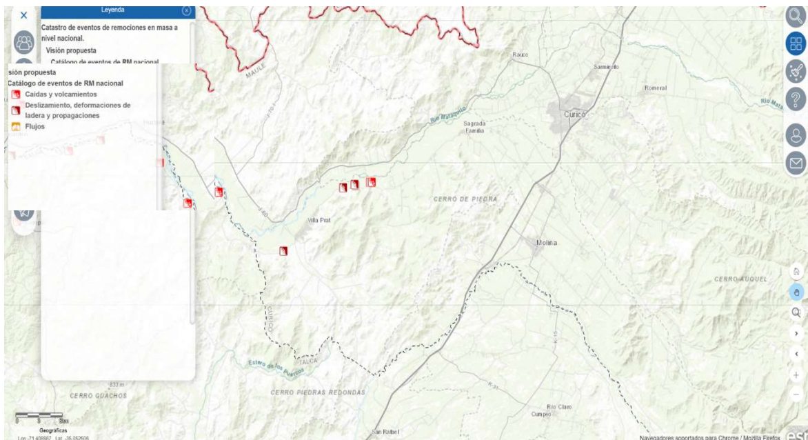
Figura 16. Catálogo de eventos de remoción en masa, comuna de Sagrada Familia
