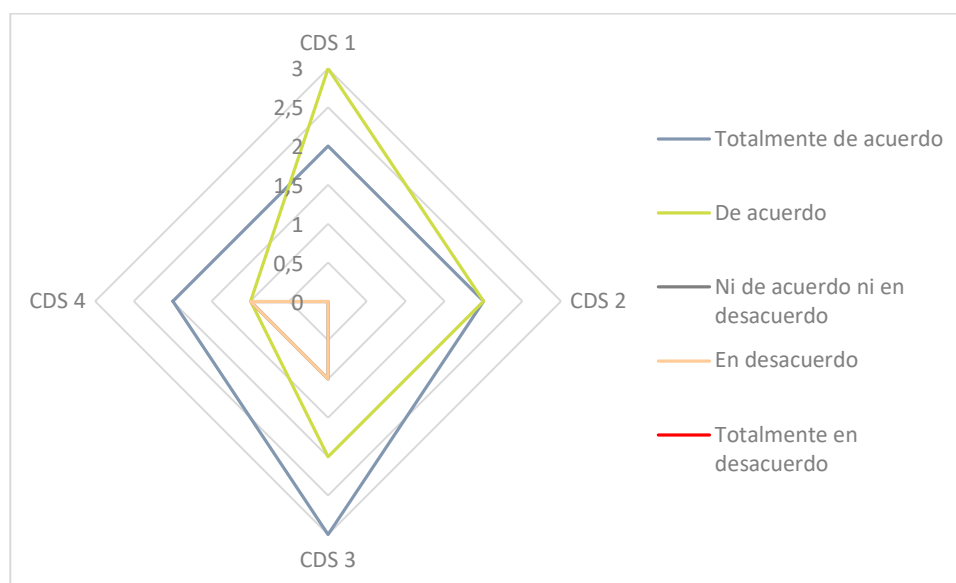
Figura 86. Niveles de acuerdo de OAE sobre Criterios de Desarrollo Sustentable
