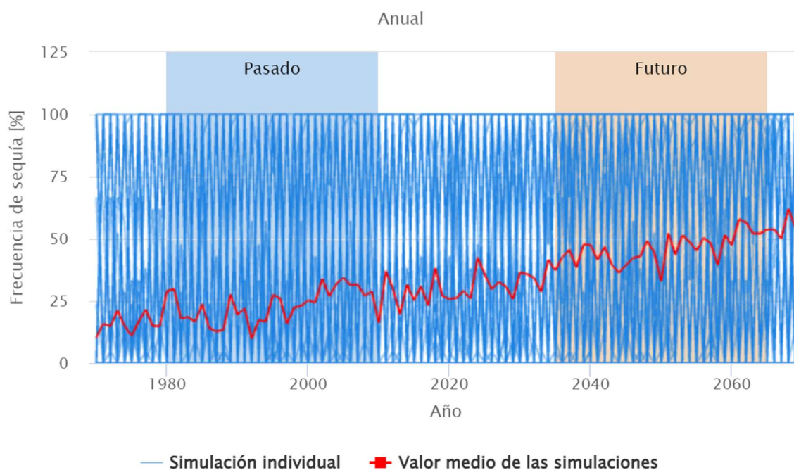
Figura 11. Frecuencia de sequía en Sagrada Familia
