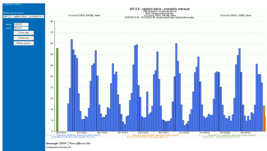
Figura 20. Promedio mensual de concentración de MP 2,5
