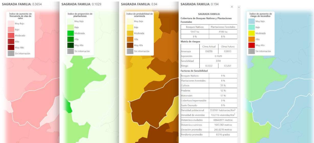
Figura 17. Riesgo de incendios forestales
