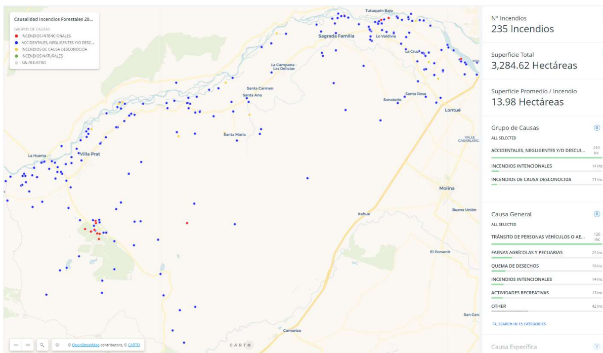
Figura 18. Causalidad de incendios forestales registrados entre el 2002 y el 2021
